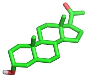
allopregnanolone
